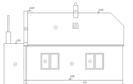
POHLED JIŽNÍ (1:50)
