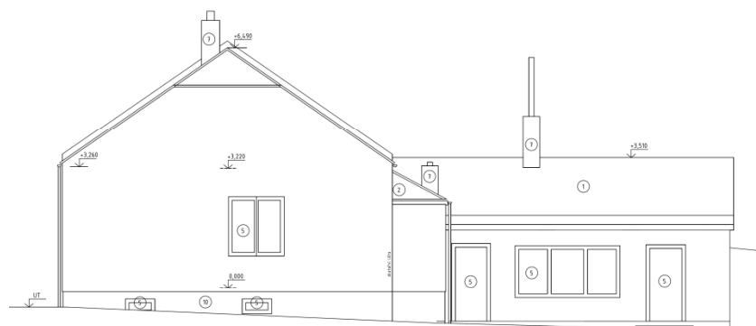
POHLED VÝCHODNÍ (1:50)
