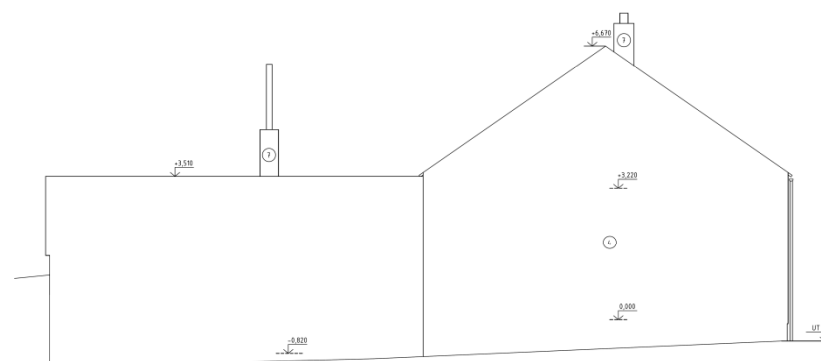
POHLED ZÁPADNÍ (1:50)
