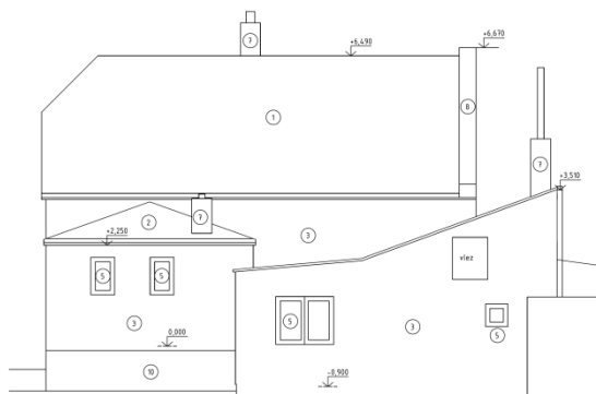
POHLED SEVERNÍ (1:50)
